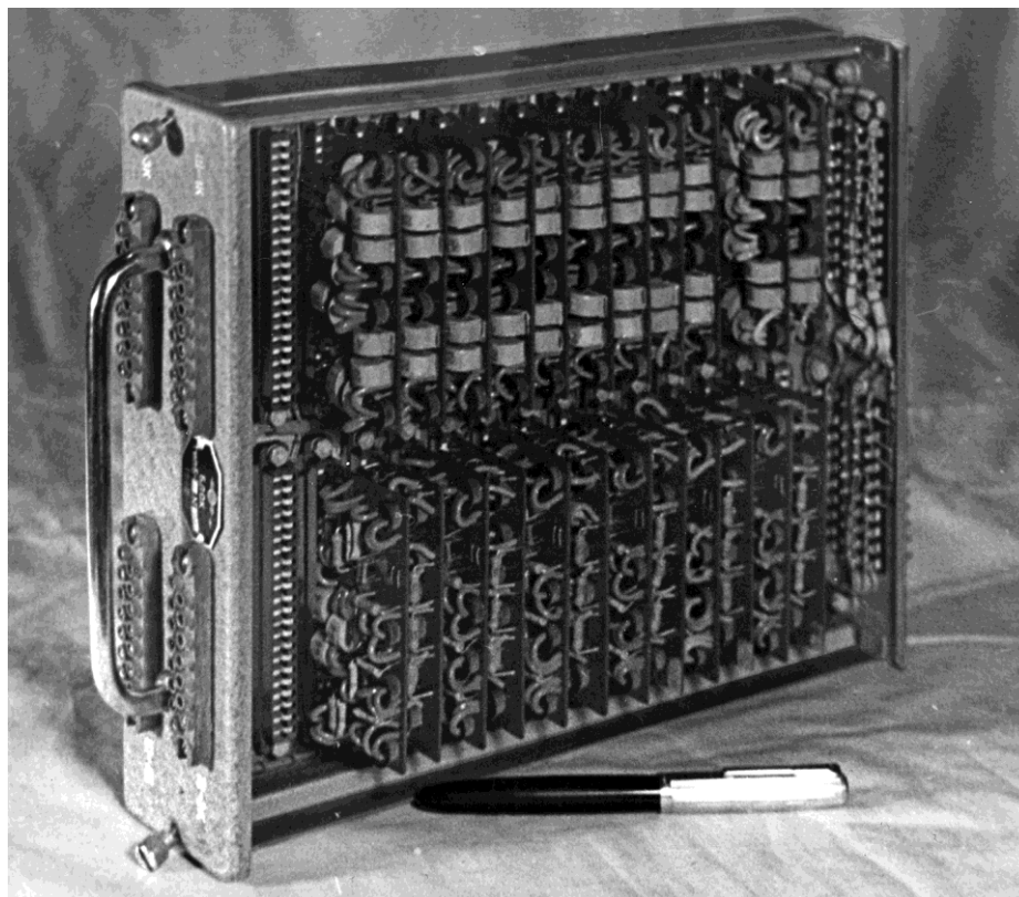
Электронный блок УМШН "Днепр" в сборе
