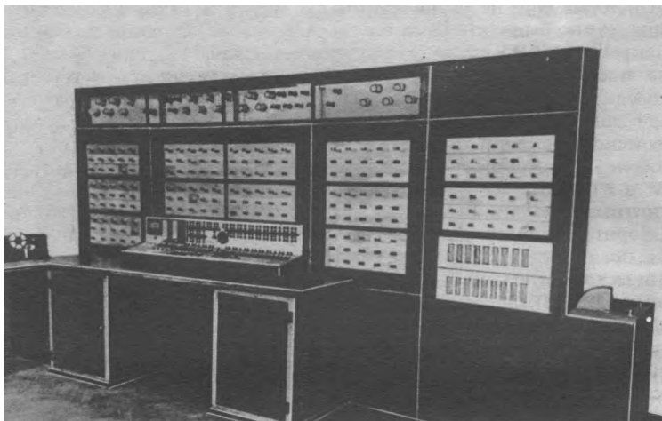
ЭВМ “Сетунь”. Опытный образец
