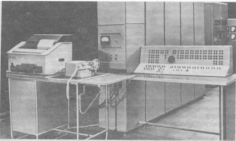
ЭВМ “Сетунь”. Промышленный образец
