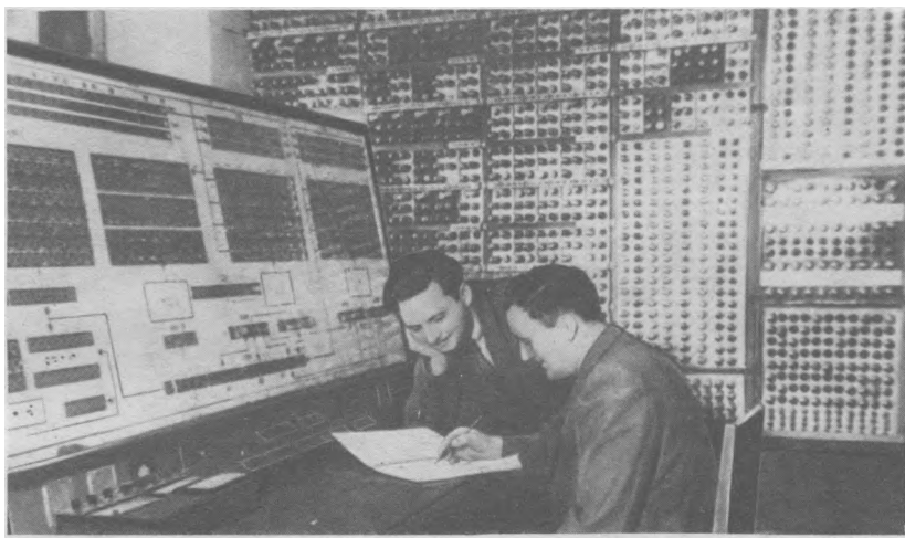
Первое детище С.А. Лебедева — МЭСМ. За пультом Л.Н. Дашевский (справа) и С.Б. Погребинский (Киев, 1951 г.)
