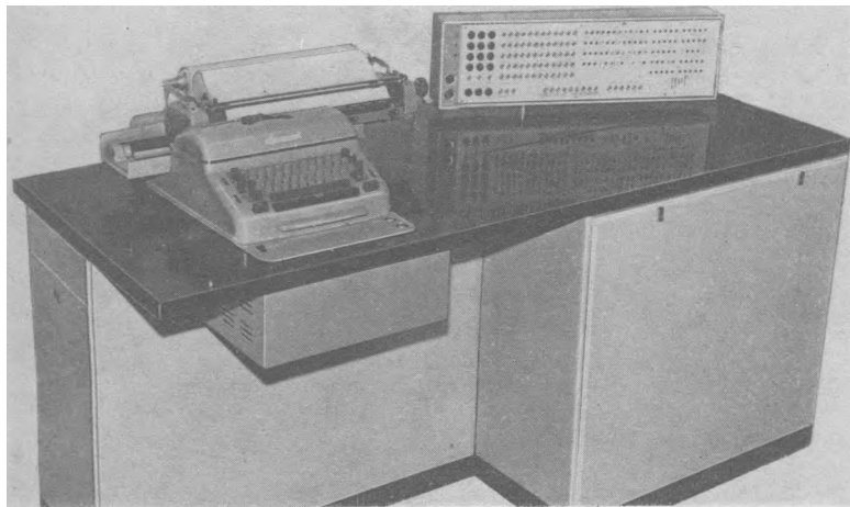
ЭВМ МИР-1
