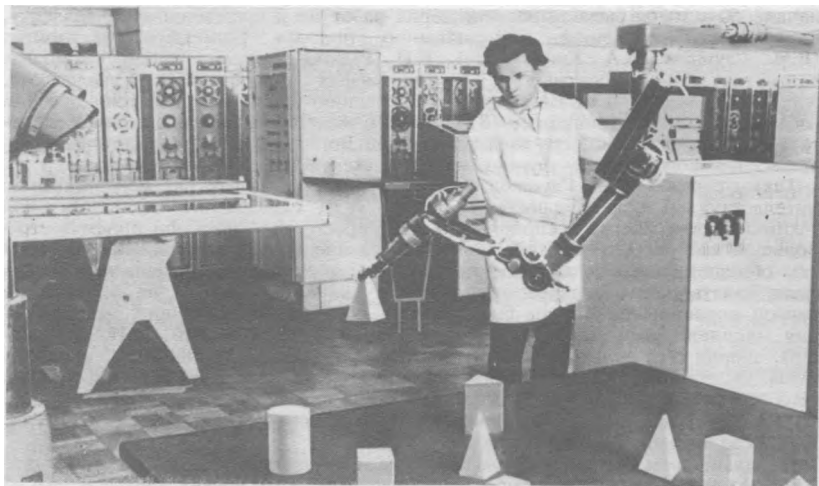
“Рука” робота, управляемая ЭВМ
