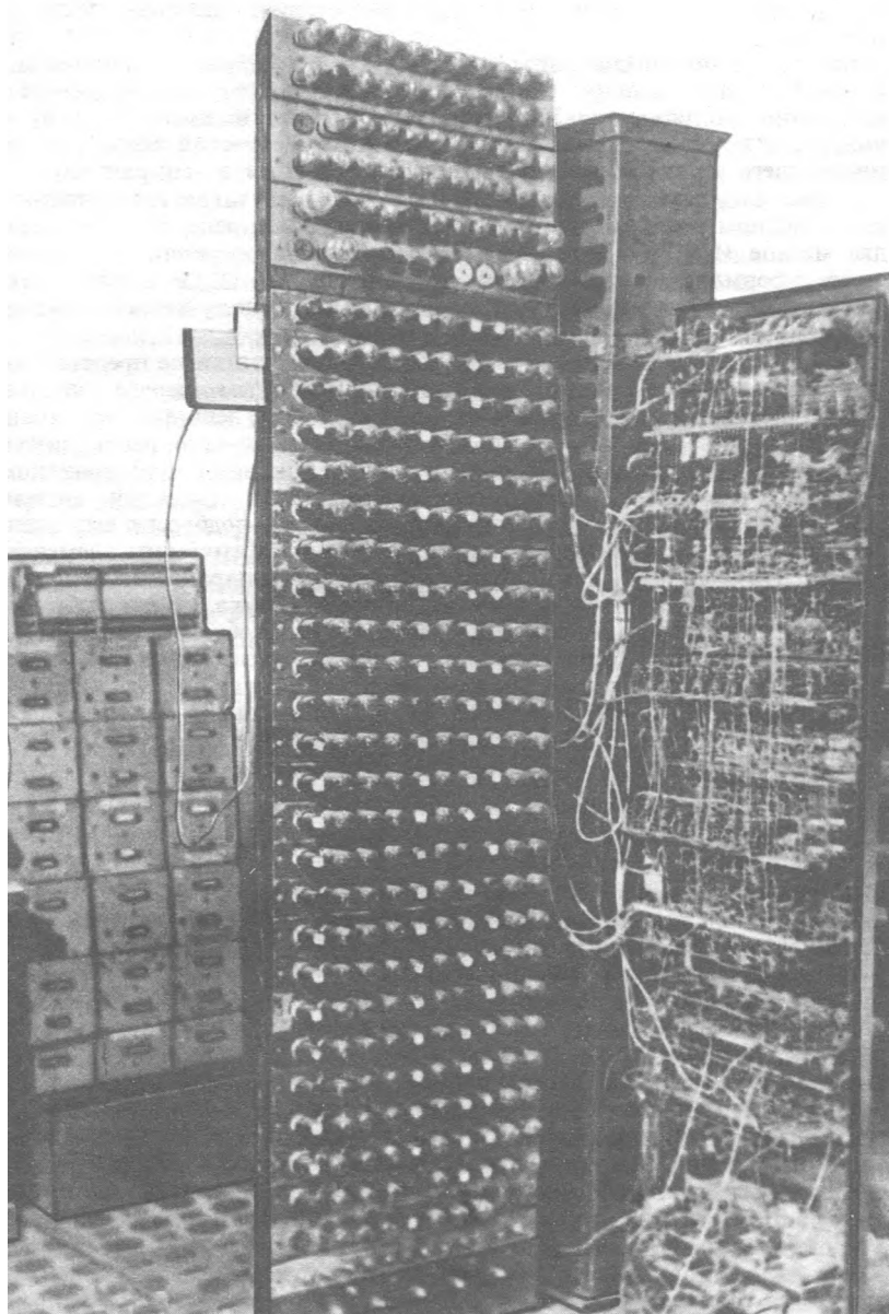
ЭВМ М-1. Общий вид
