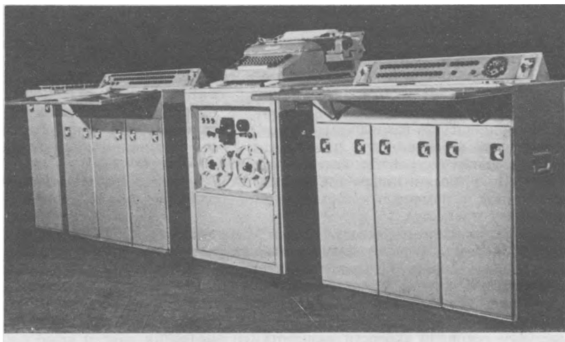
Управляющая машина широкого назначения “Днепр” (УМШН)
